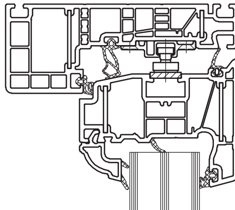
FIG. 2 VANDRET SNIT
