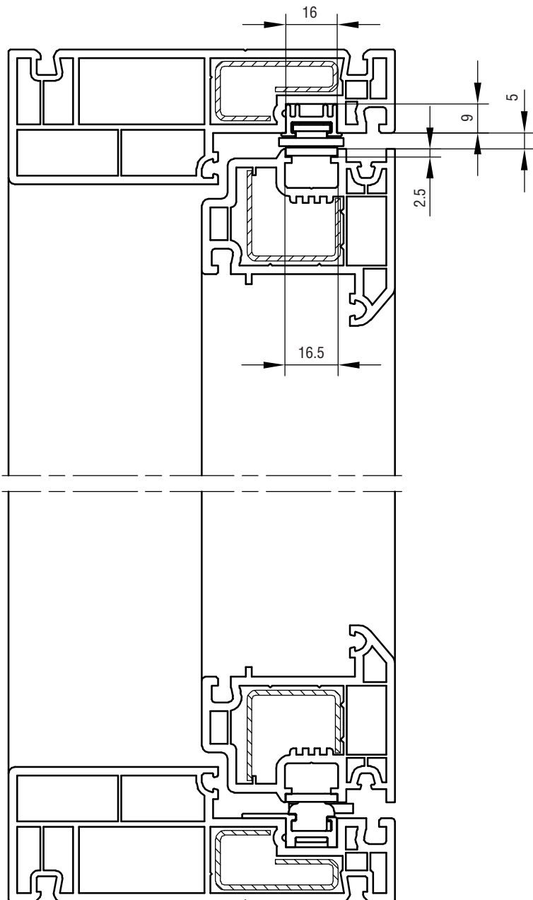
FIG. 1 LODRET SNIT
