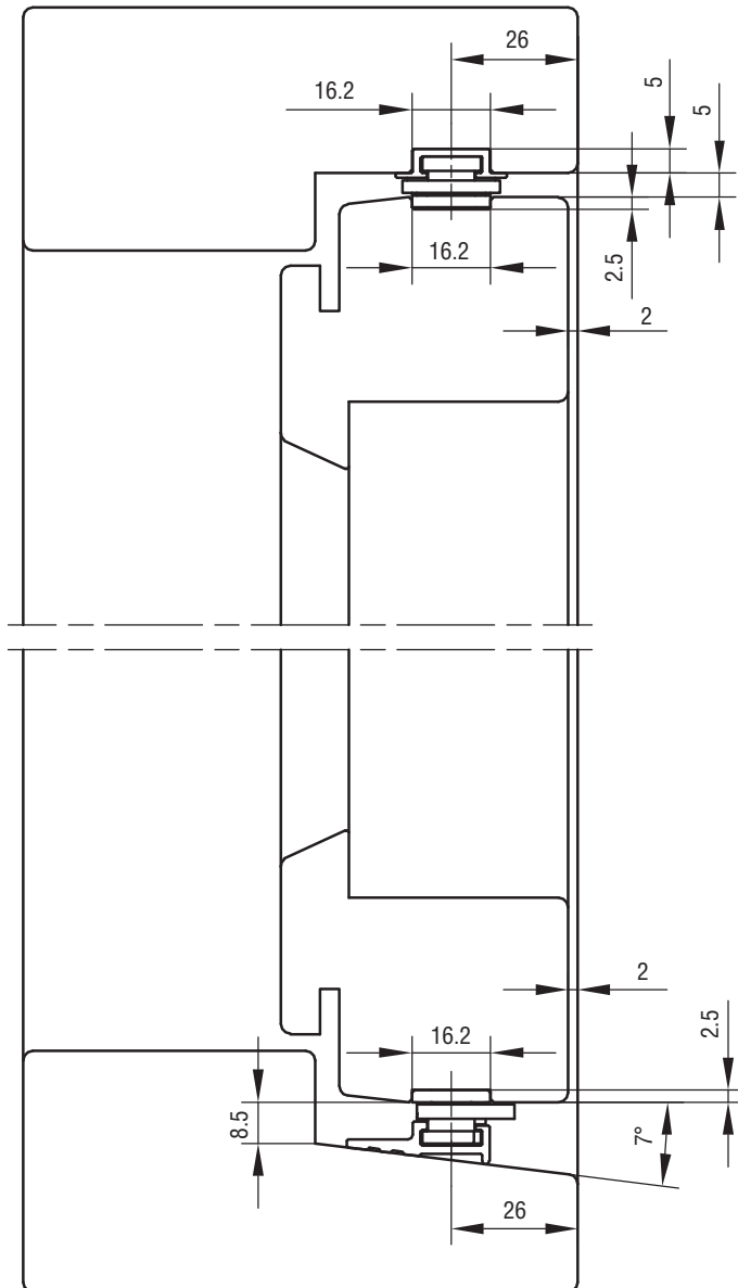
FIG. 1 LODRET SNIT
