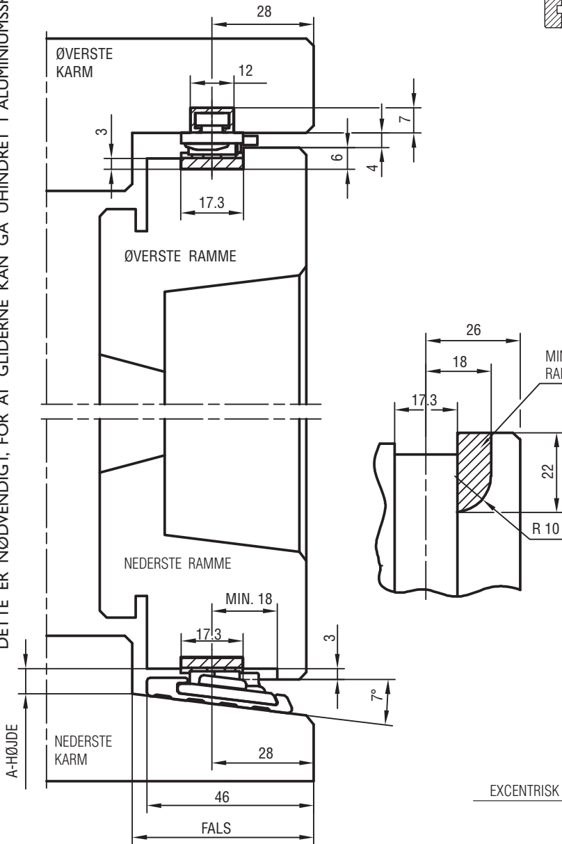
FIG. 1 LODRET SNIT
